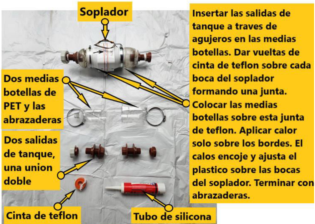
DESPIECE DEL SOPLADOR
